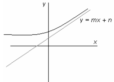
Asíntota oblicua
